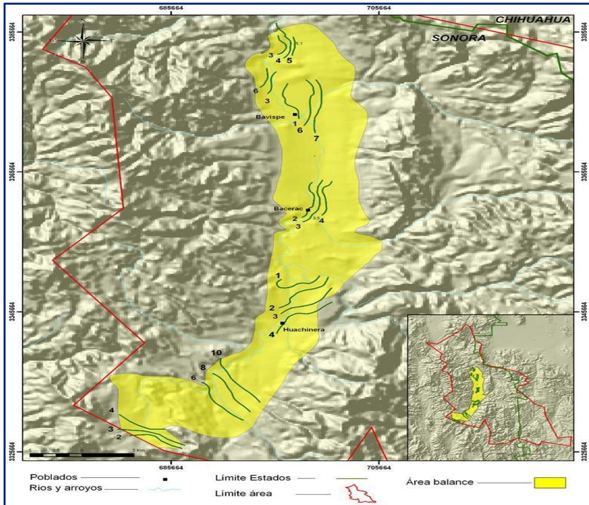
Figura 4. Profundidad al Nivel Estático en m (2008) y zona de balance
