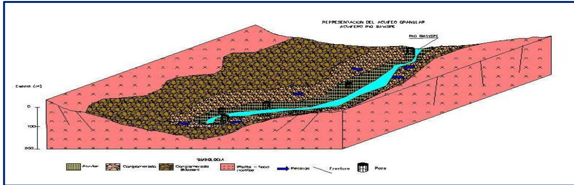
Figura 3. Modelo conceptual de funcionamiento acuífero
