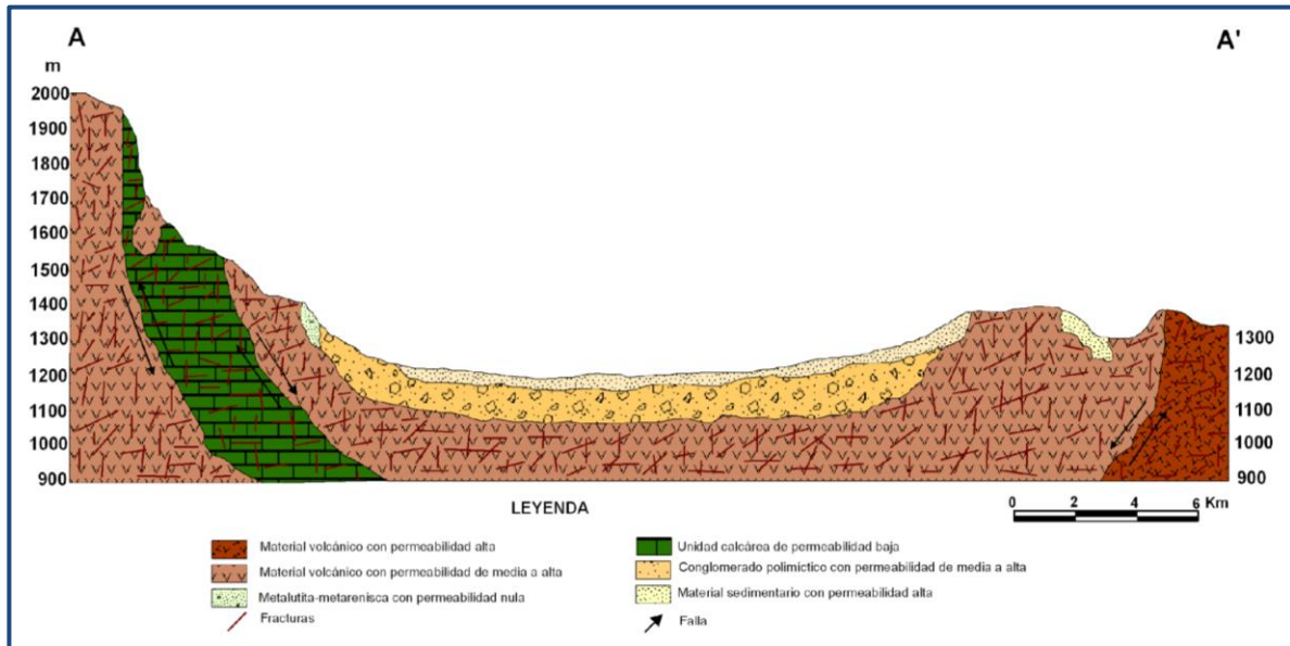
Figura 3. Sección Hidrogeológica A-A'
