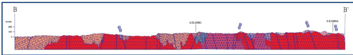
Figura 3. Sección geológica
