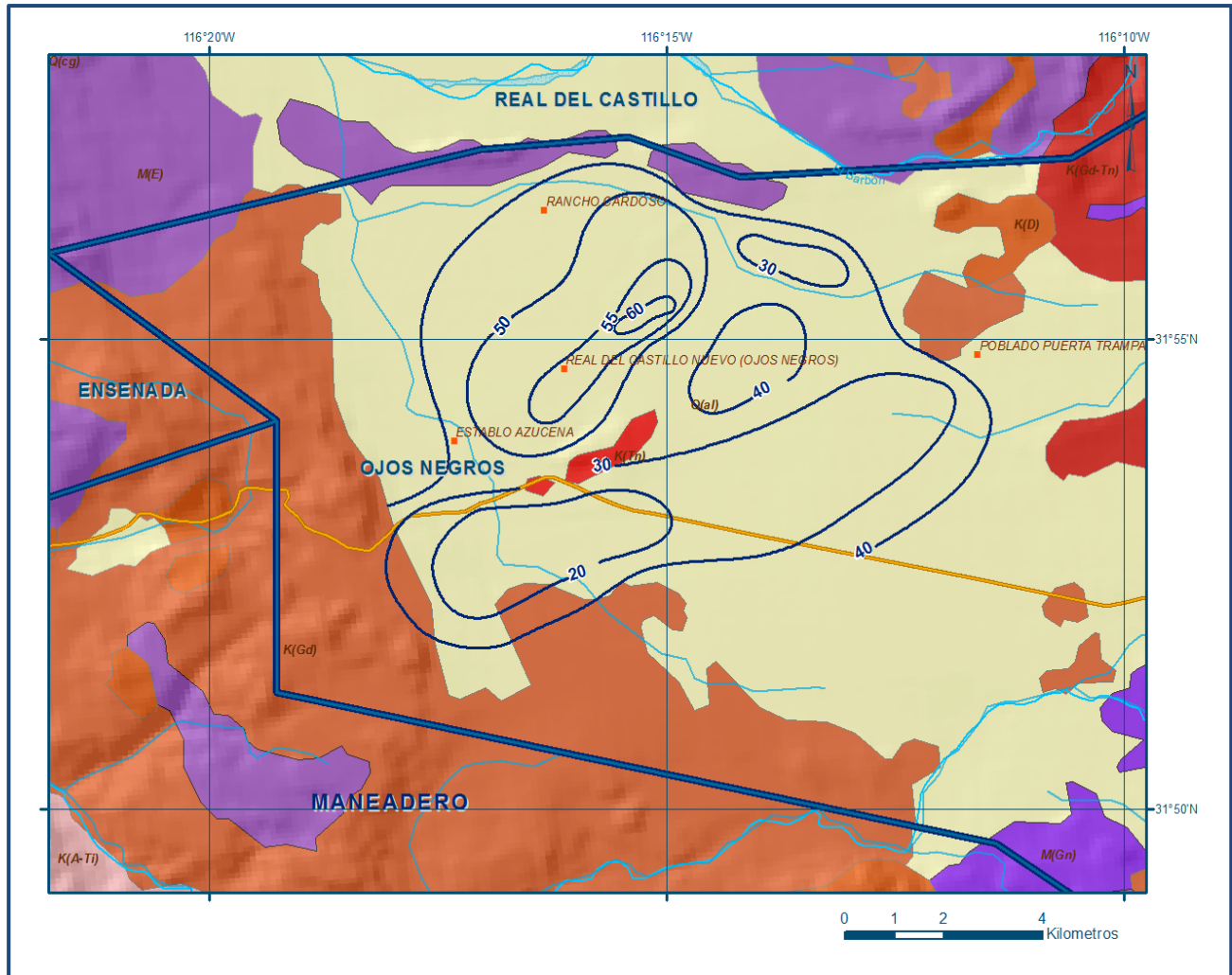
Figura 4. Profundidad al nivel estático en m (2013)
