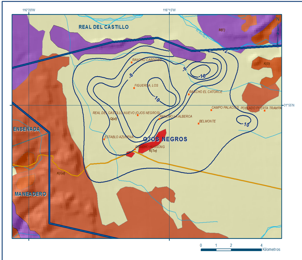
Figura 6. Evolución del nivel estático en m (2008-2014)
