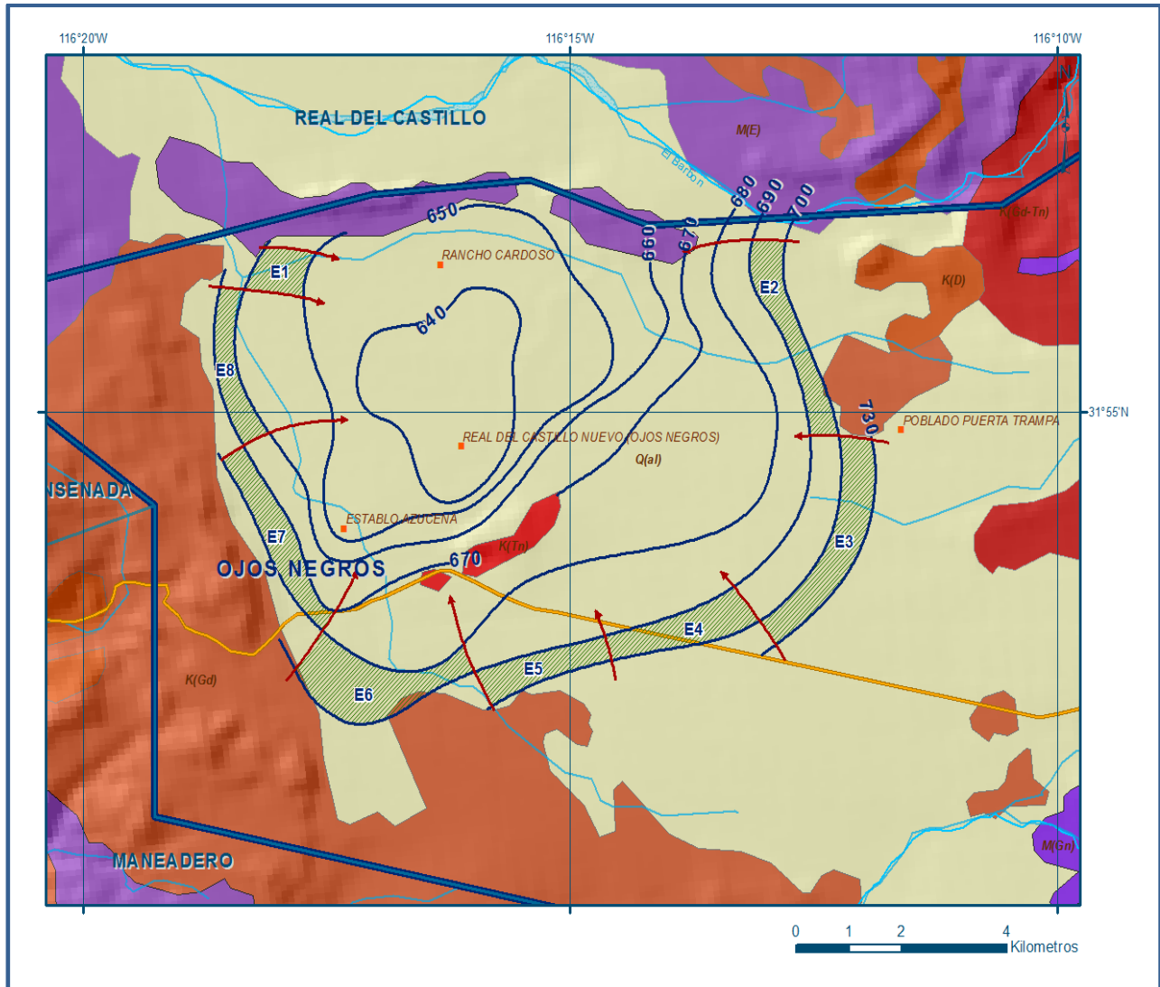
Figura 5. Elevación del nivel estático en msnm (2013)
