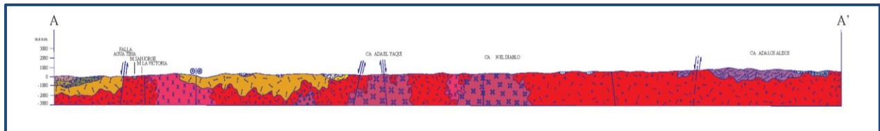
Figura 3. Sección geológica
